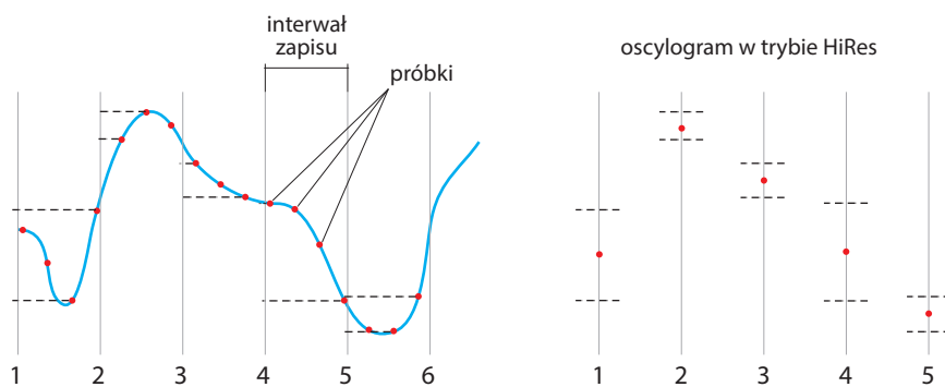
Rysunek 5. Zasada pracy układu akwizycji w trybie HiRes
