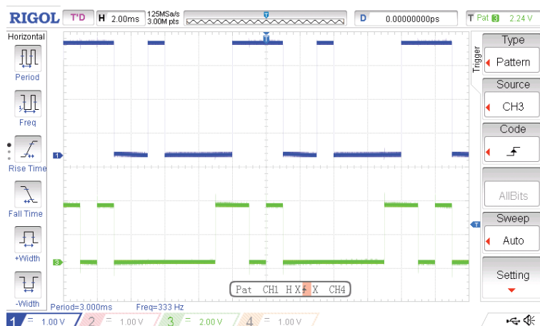
Rysunek 7. Wyzwalanie wzorcem
