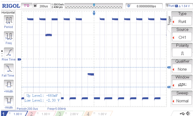
Rysunek 9. Wyzwalanie Runt
