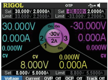
DP831A GUI
